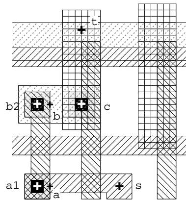
(d) Our result
